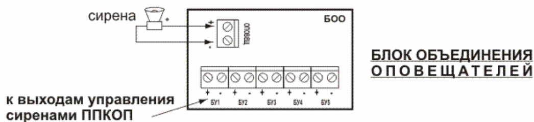
Рис. 6.3. Схема подключения одного звукового оповещателя (сирены) к нескольким приборам "grand МАГИСТР"
