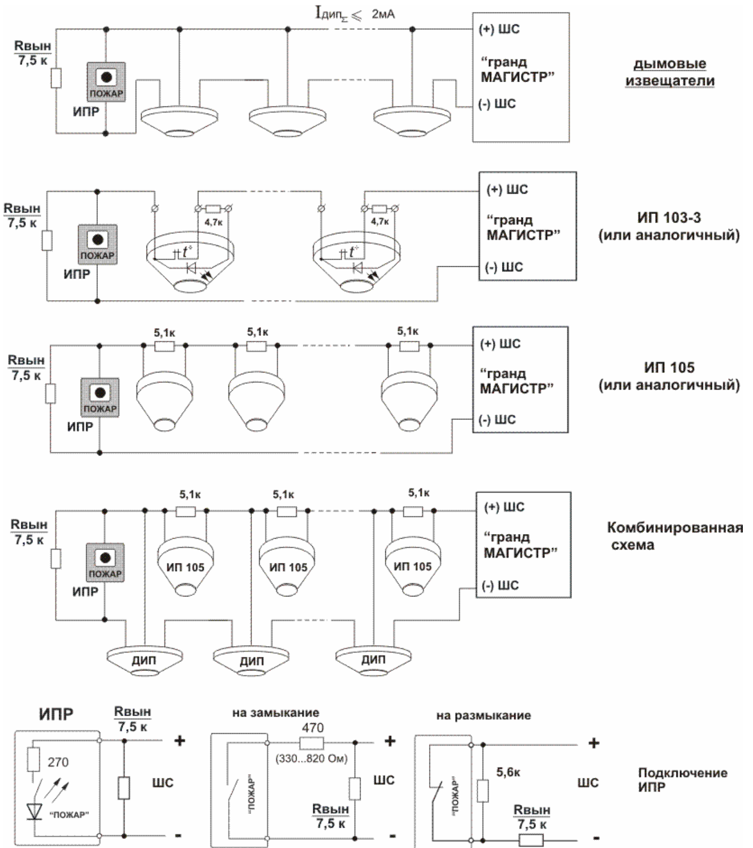
Рис. 4.3. Организация однопорогового шлейфа пожарной сигнализации
